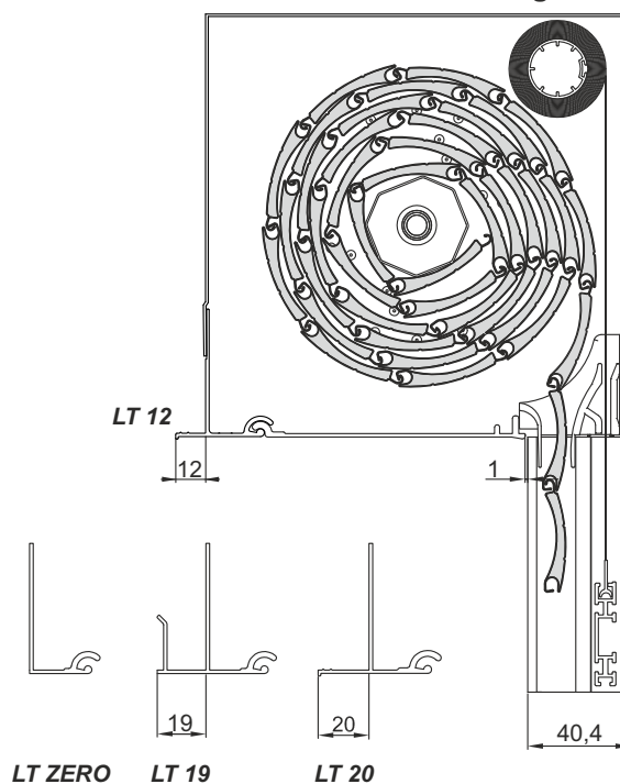
Rollladen IT2000® mit Insektenschutzgitter
